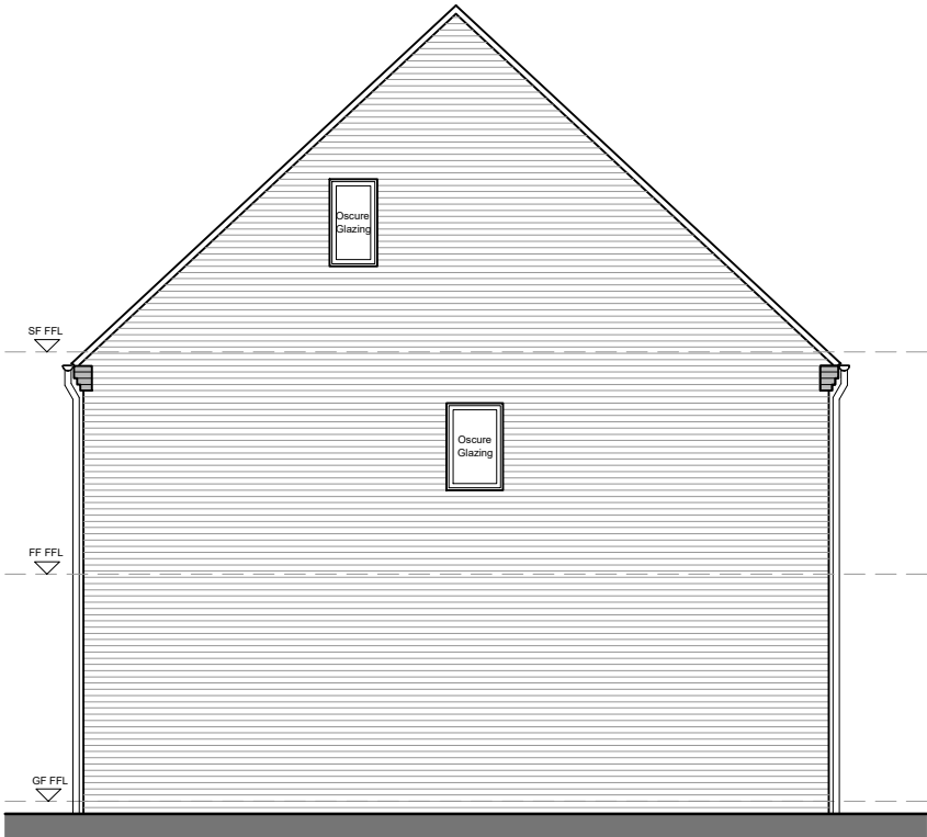
R.H.S. Elevation
