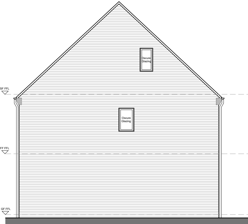
L.H.S. Elevation
