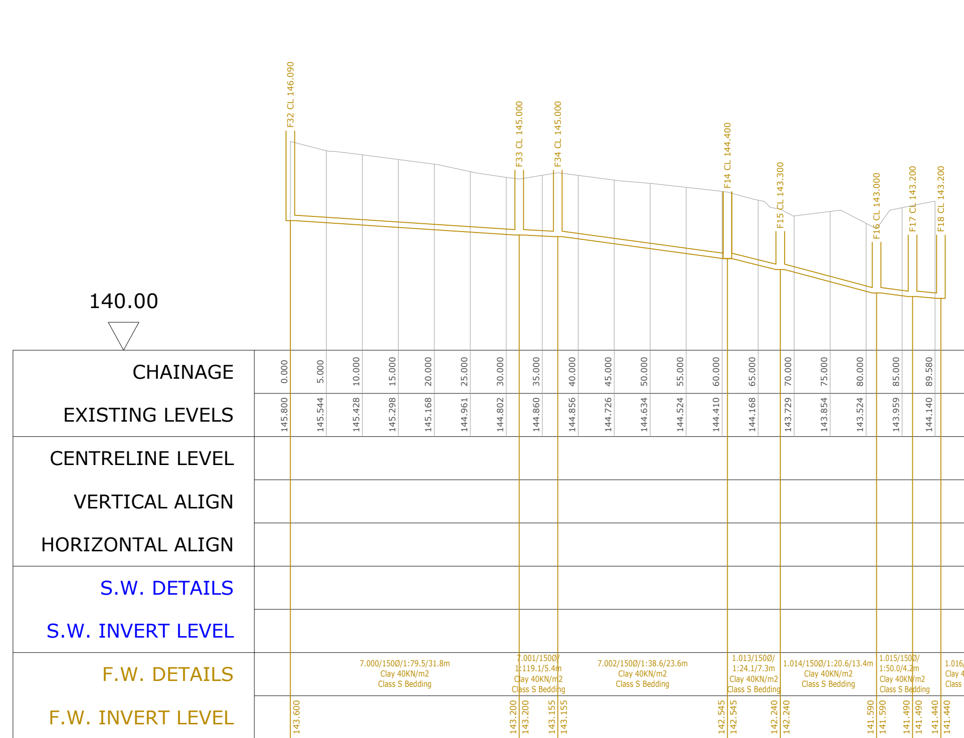
F32-F18 Horiz. 1:500 Vert. 1:100
