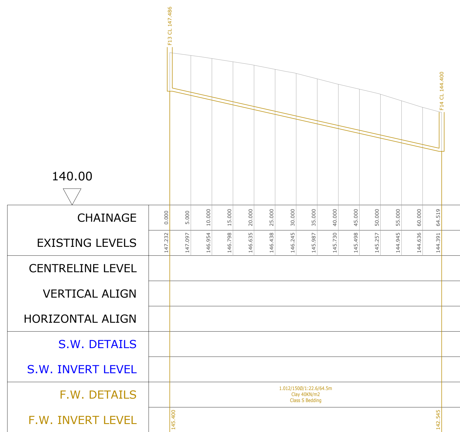
F13-F14 Horiz. 1:500 Vert. 1:100
