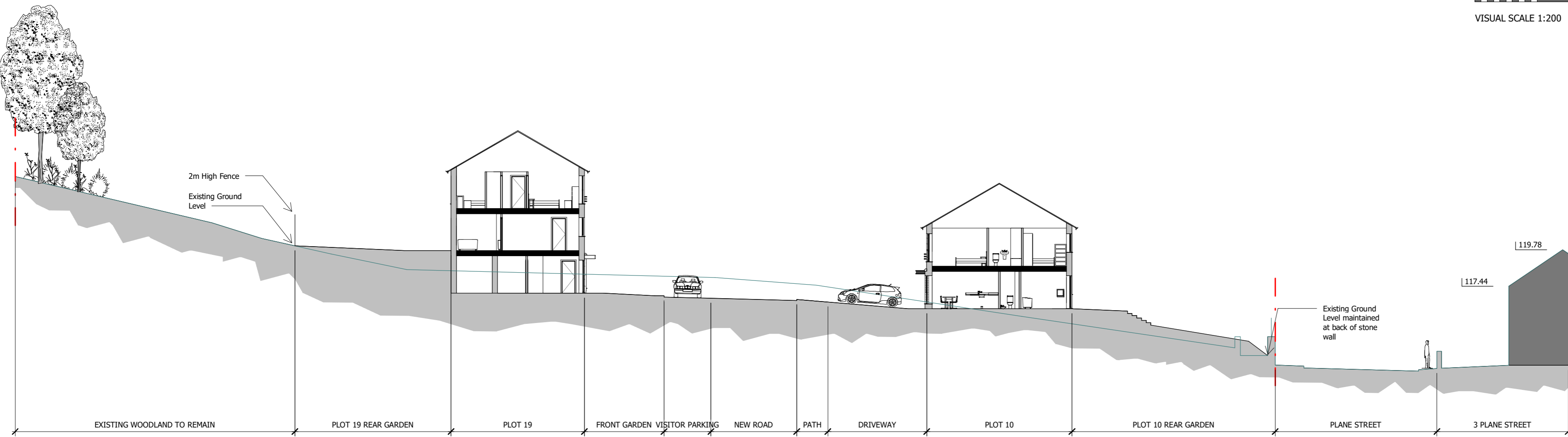
Site Section A 1 : 200
