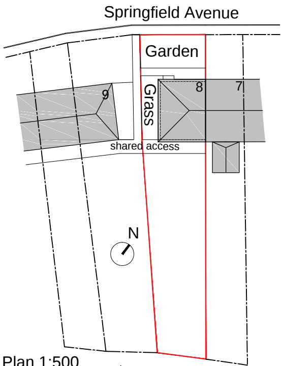
Site Plan 1:500
