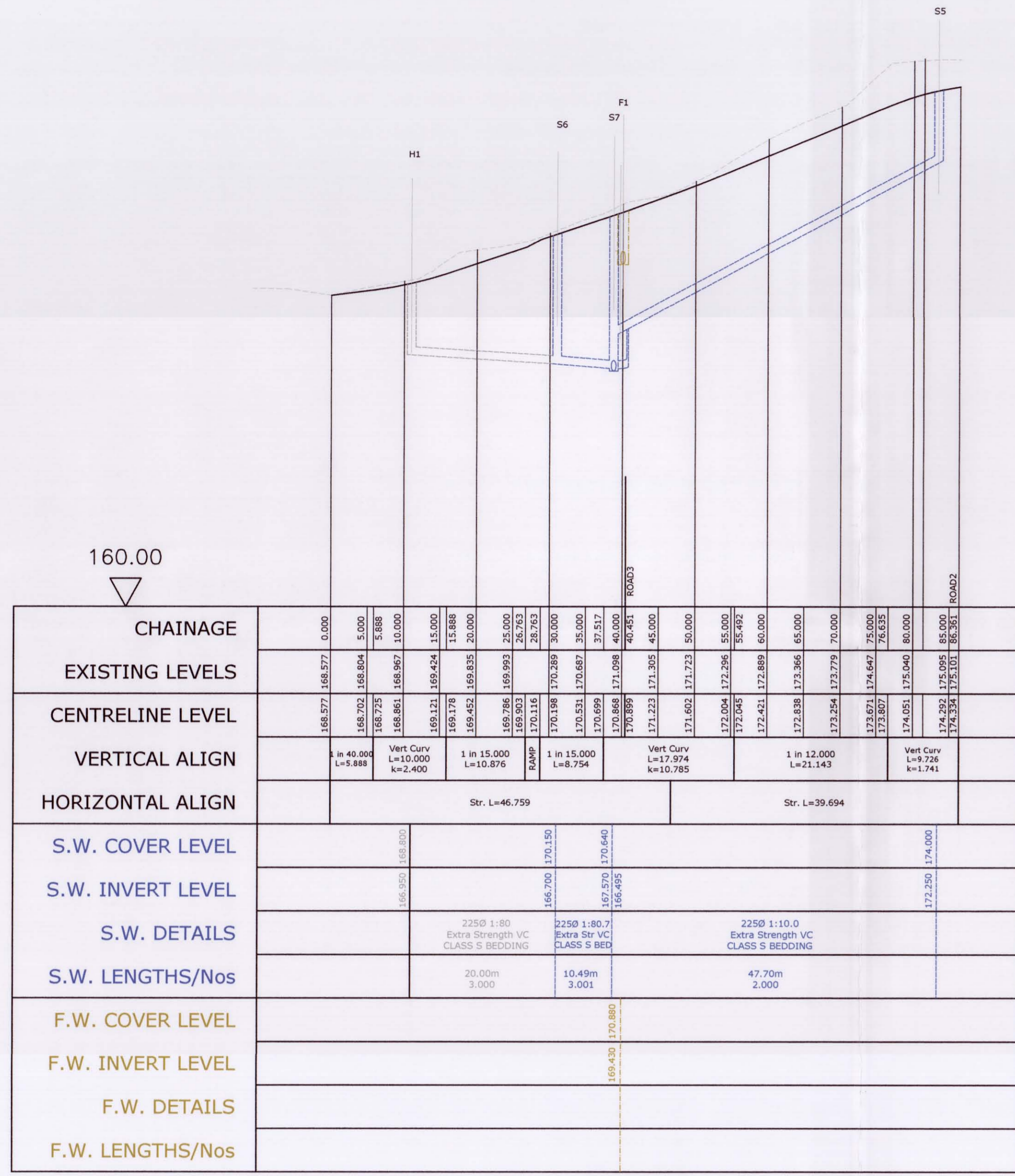
Road 1 Horiz. 1:500 Vert. 1:100
