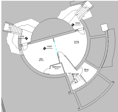
00-Basement Scale 1 : 100
