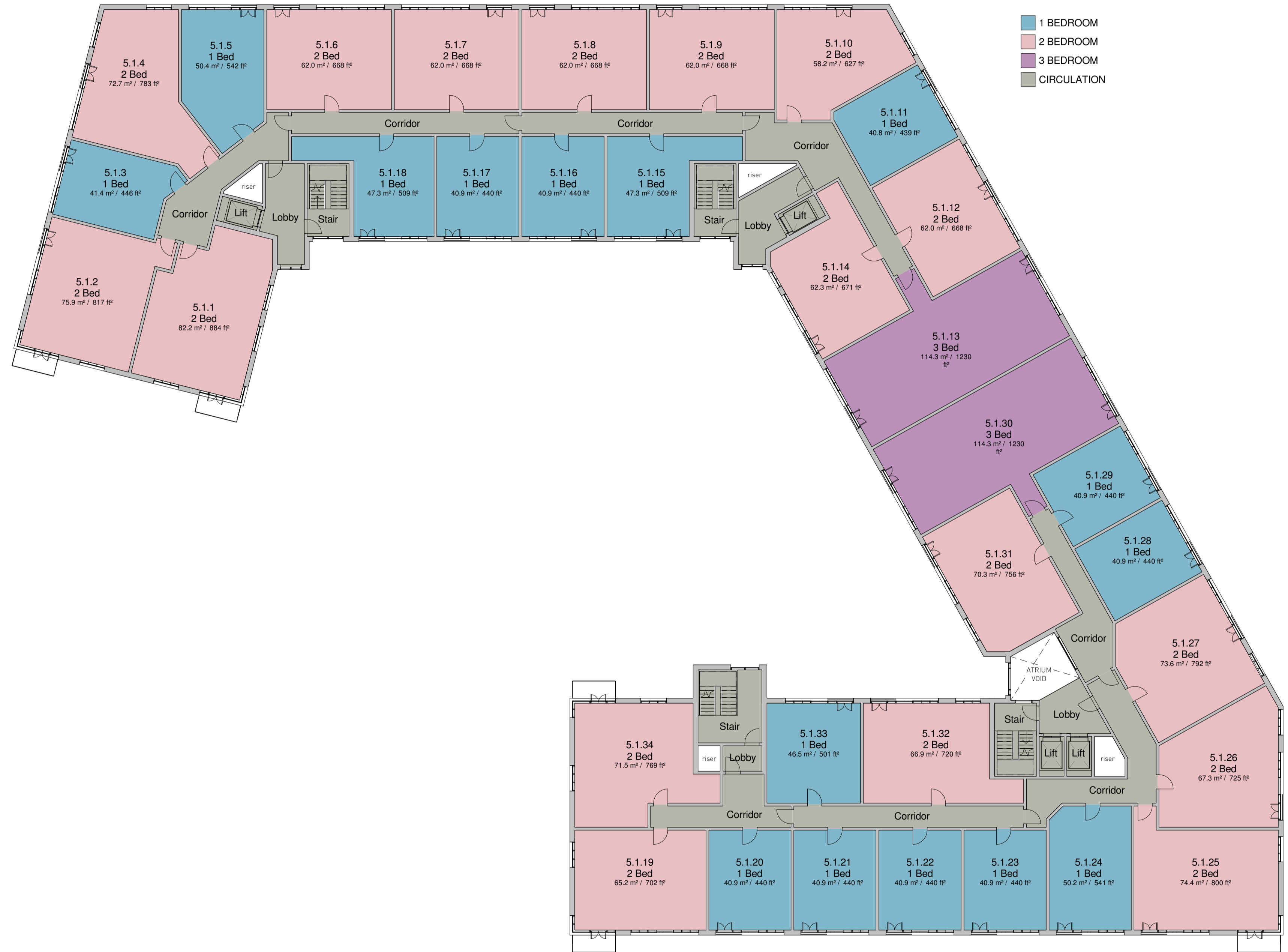
Levels 01-03 GA Plan 1 : 200
