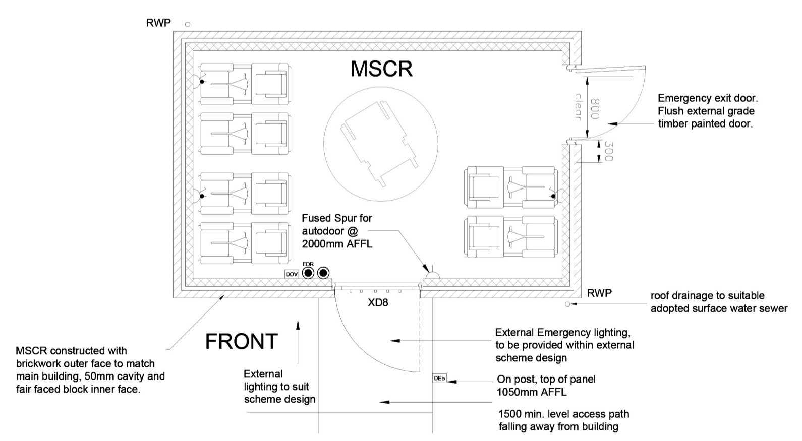
1 MSCR Layout 1:50
