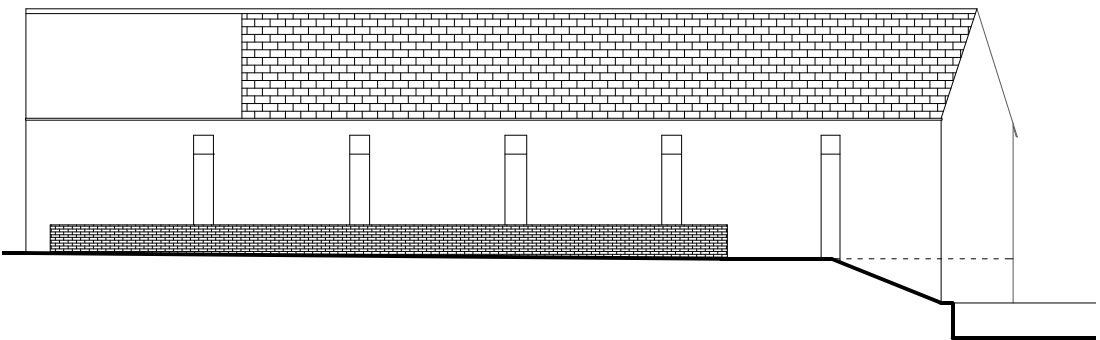
SE elevation
