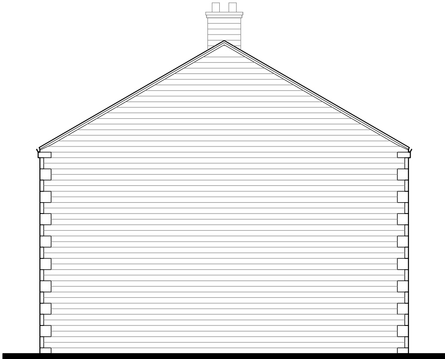
R.H. SIDE ELEVATION
