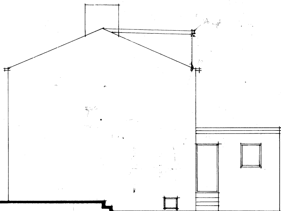
SIDE 1:100
