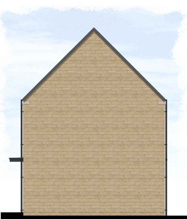
Right Elevation
