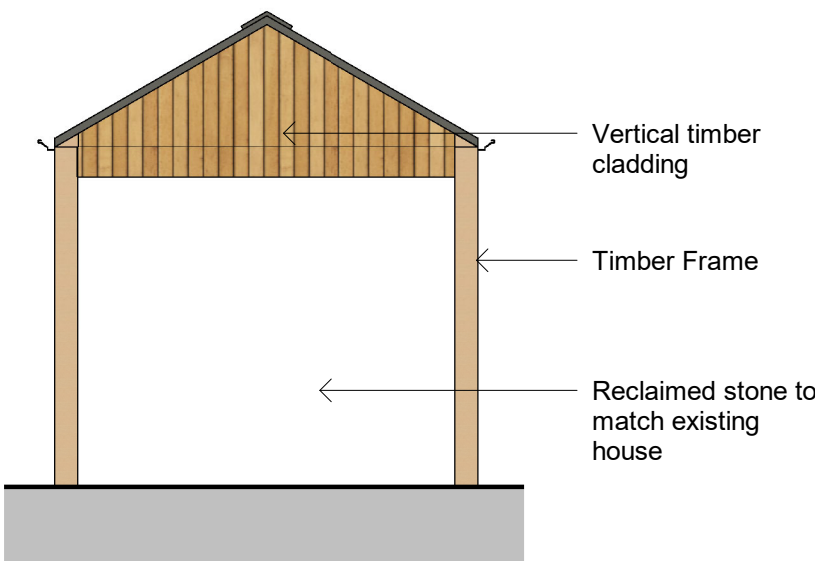
Elevation - A
