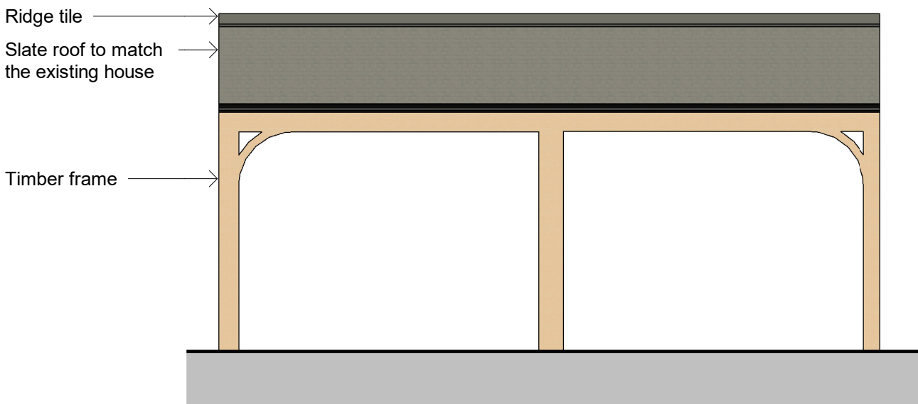
Elevation - B
