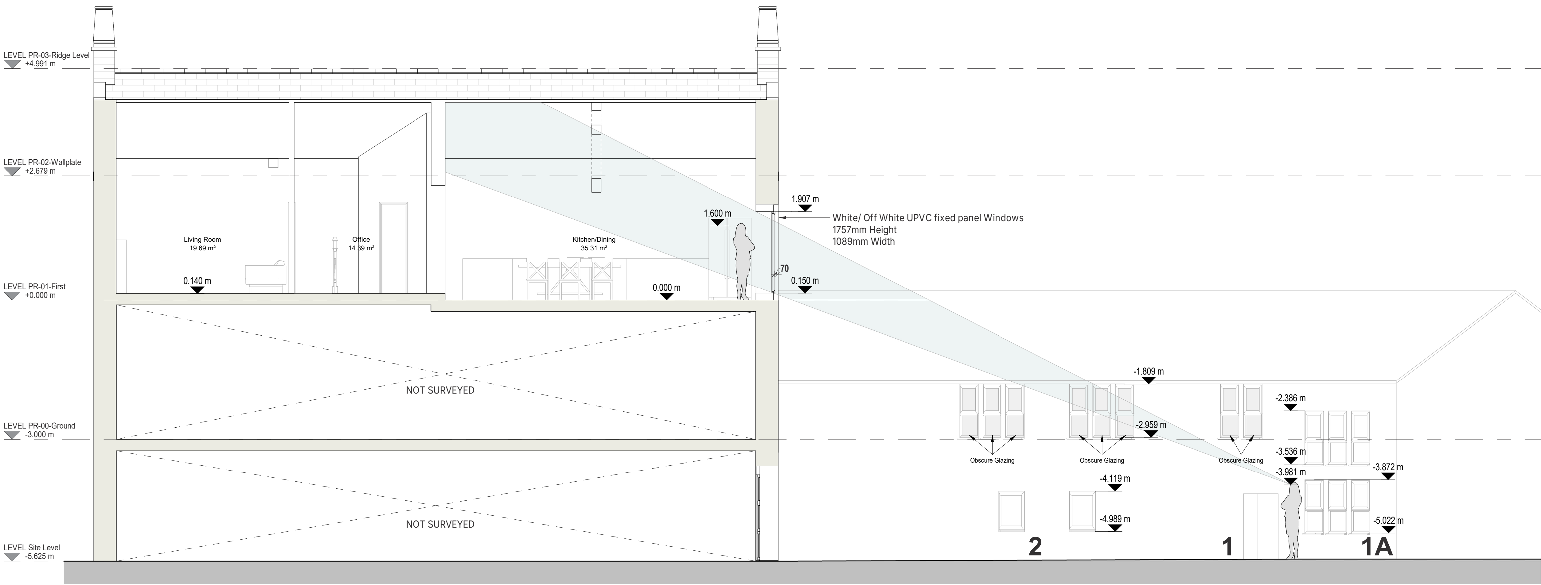
Section 1 1 : 50
