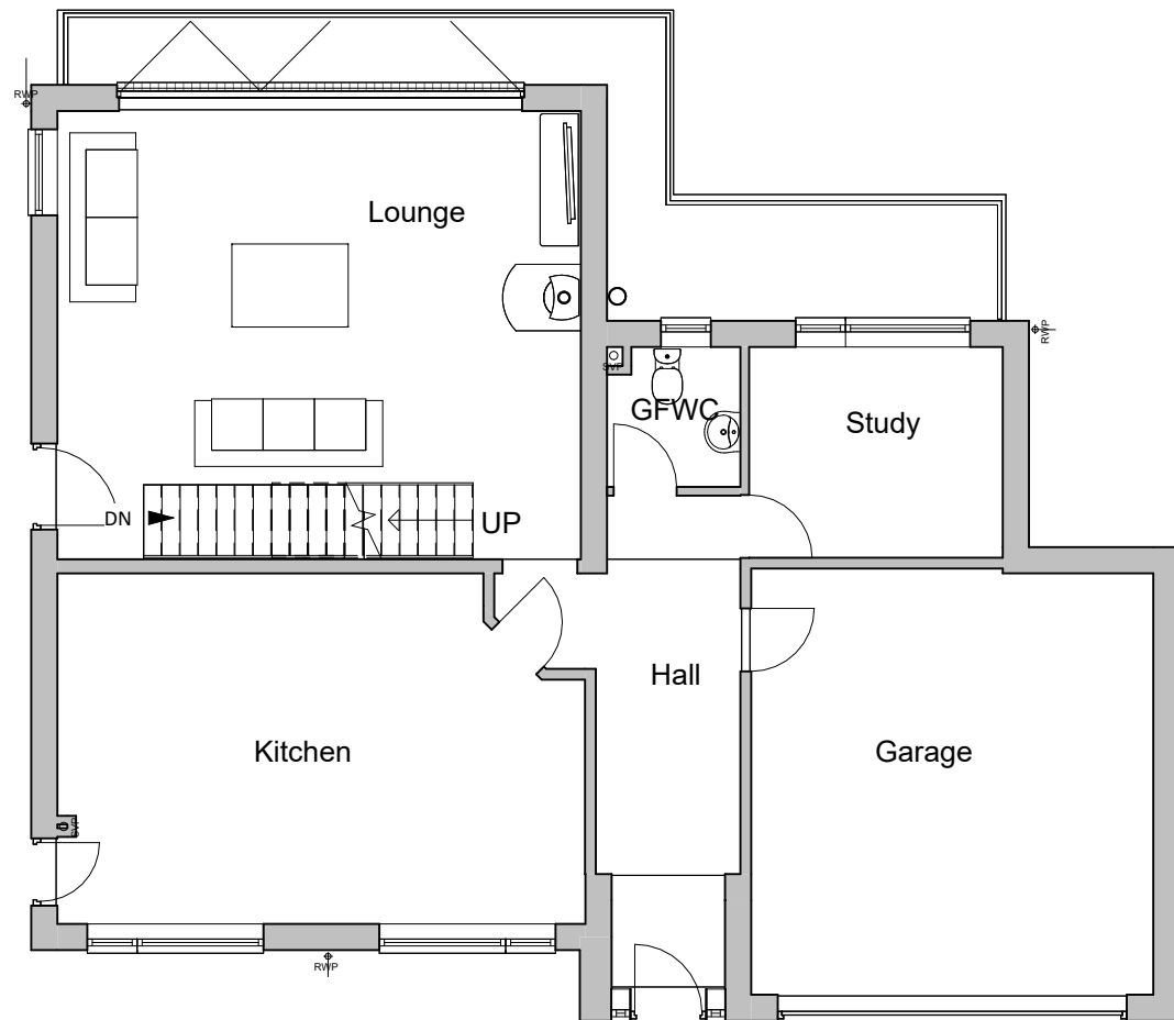
2 02b GF Existing 1 : 100
