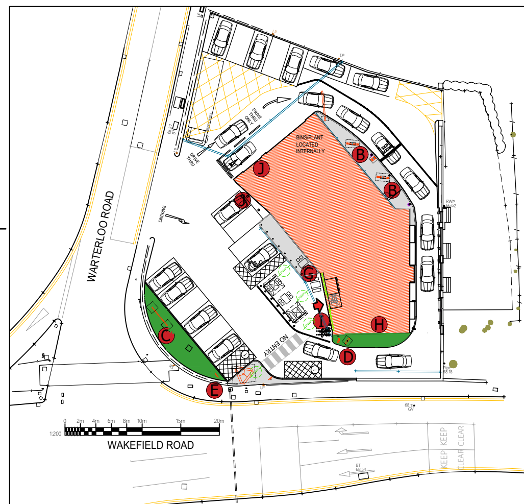
SITE PLAN 1:500
