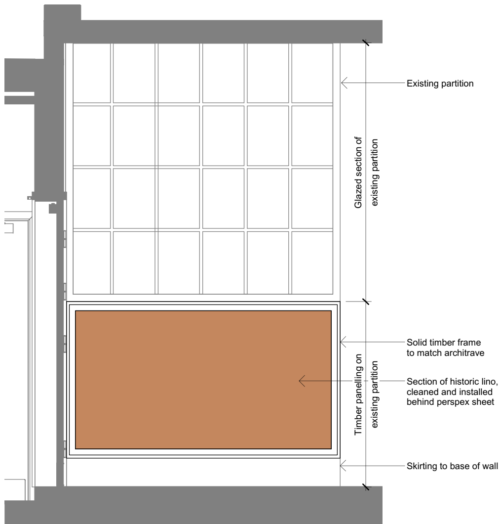
1:20 Elevation
