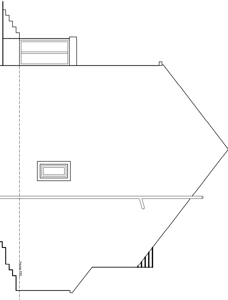
E101 Existing Left Elevation 1:100
