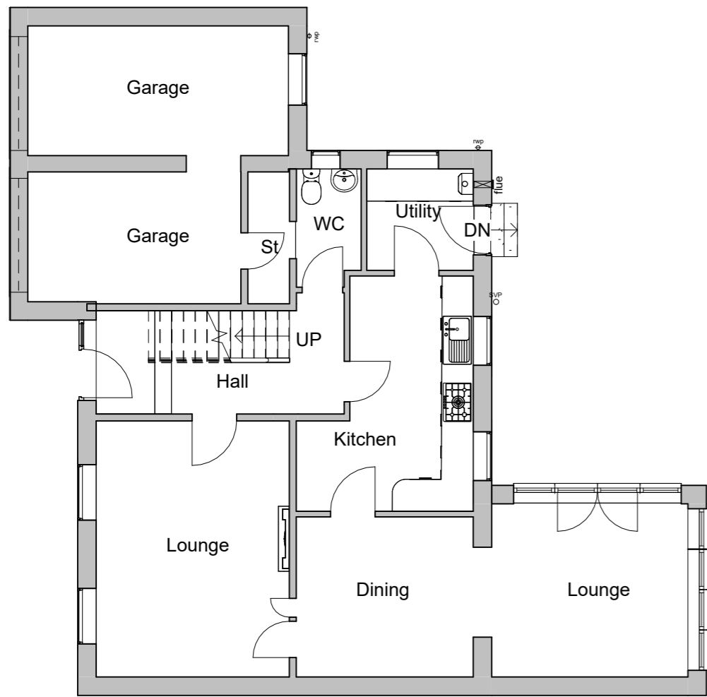
1 02a GF Existing 1 : 100
