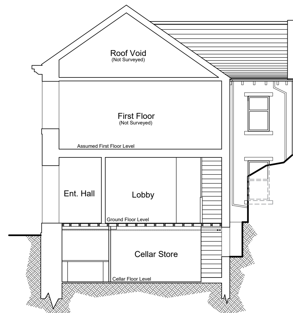
Section A-A
