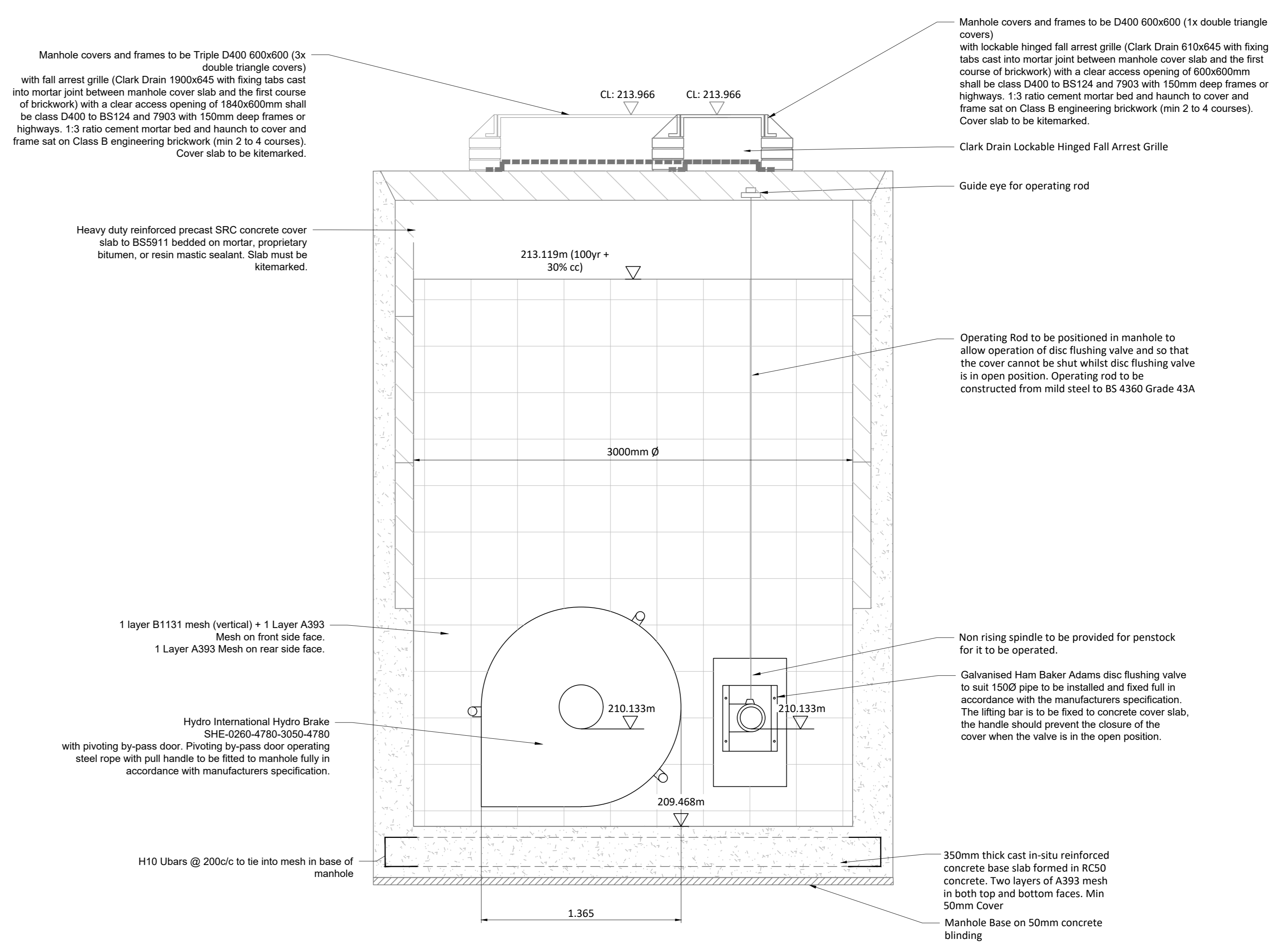
Section A-A Scale 1:20
