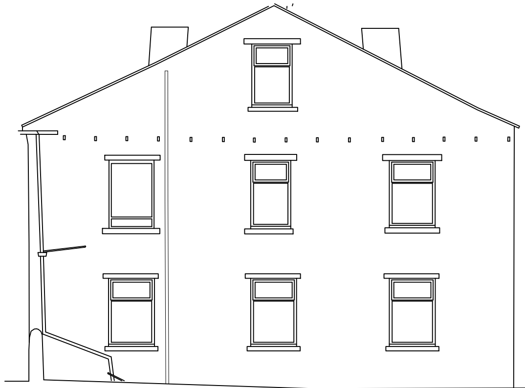
ELEVATION A
