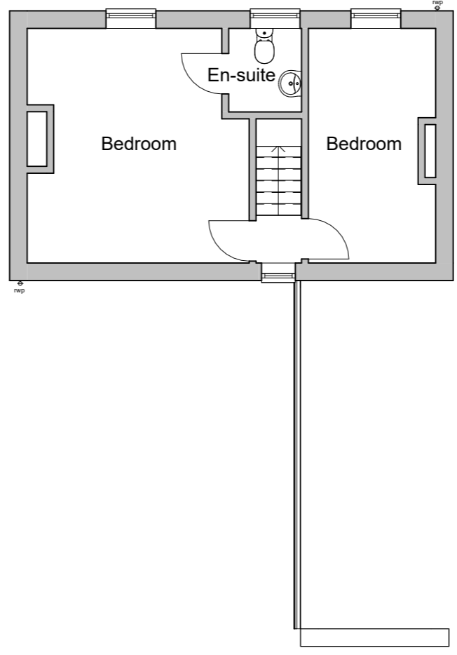
2 03a FF Existing 1 : 100
