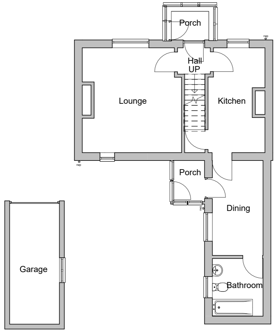
1 02a GF Existing 1 : 100
