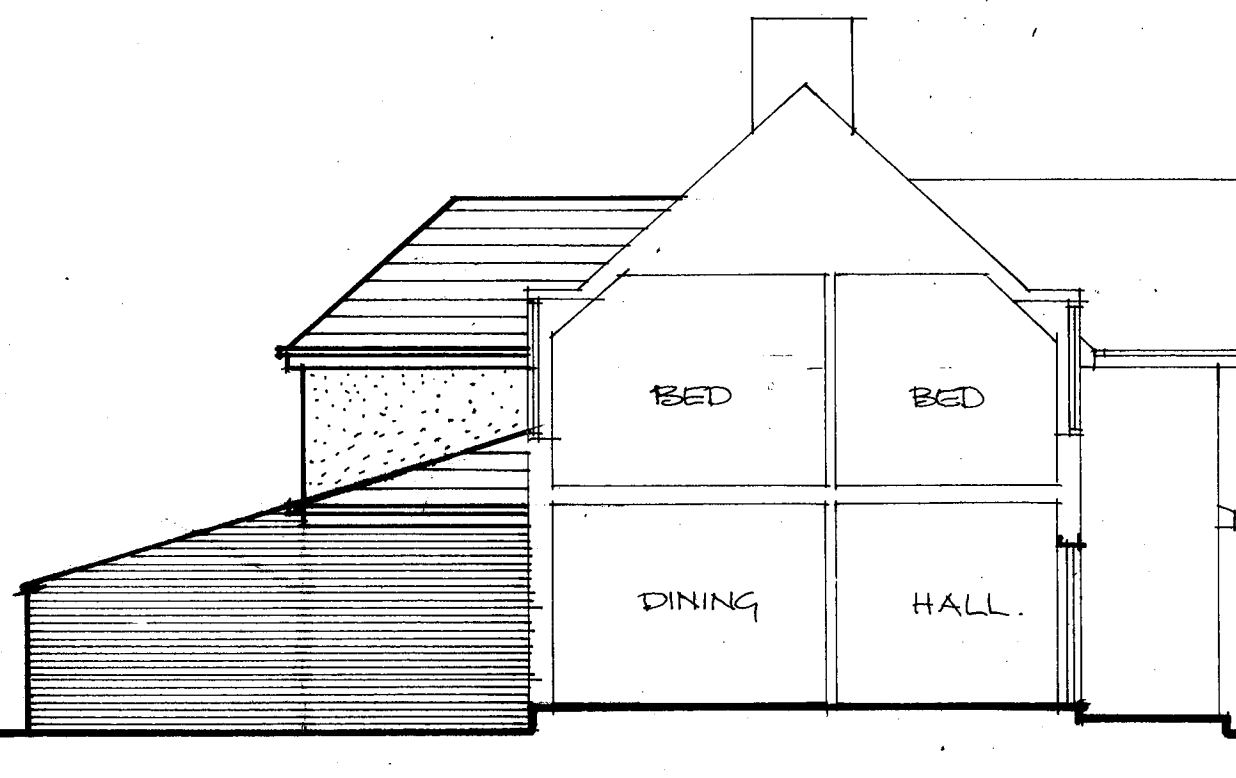
SIDE 1:100
