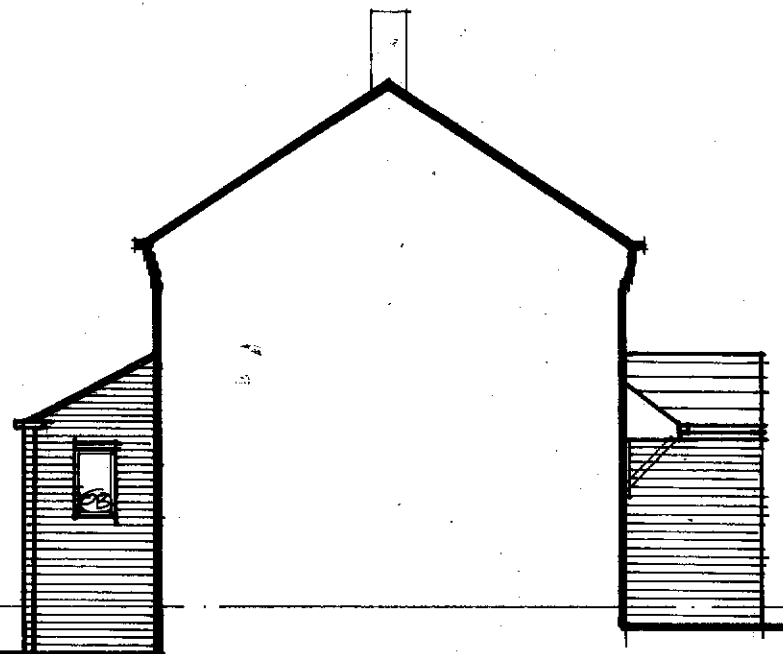
SIDE 1:100
