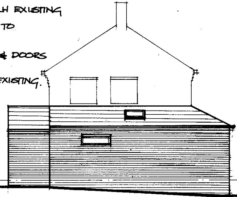
SIDE 1:100
