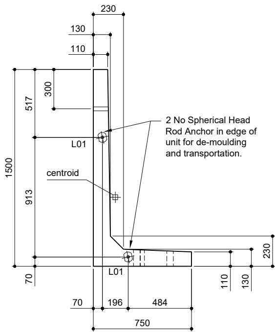
Elevation A-A
