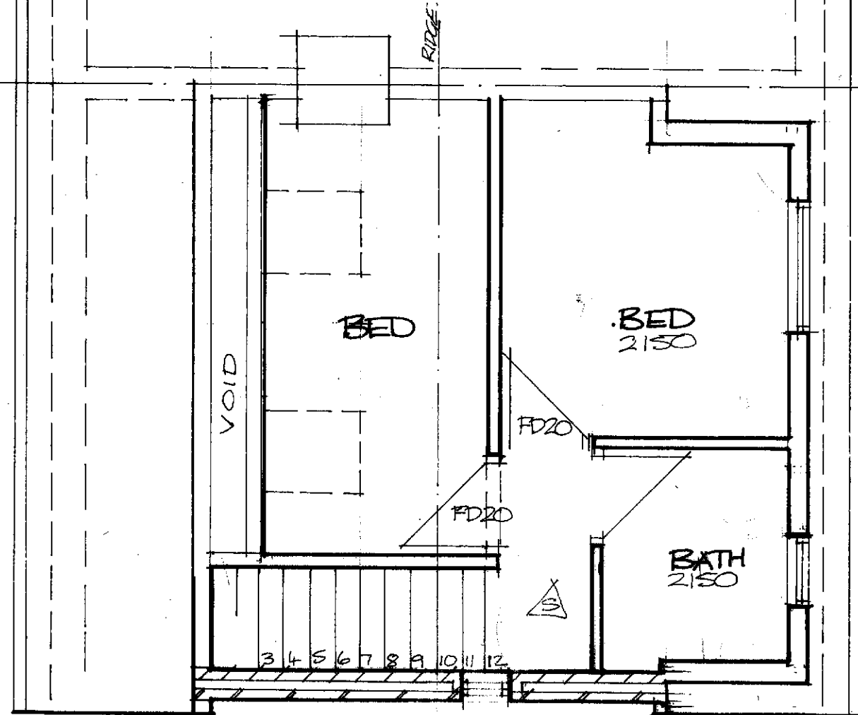
LOFT 1:50
