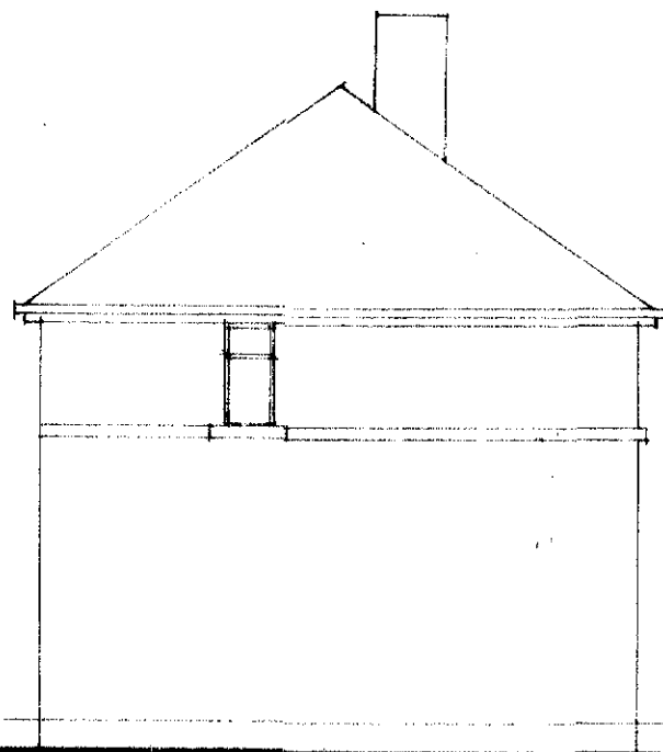
SIDE 1:100
