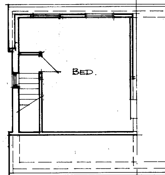
LOFT 1:100
