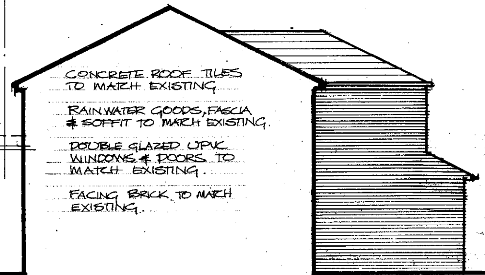
SIDE 1:100
