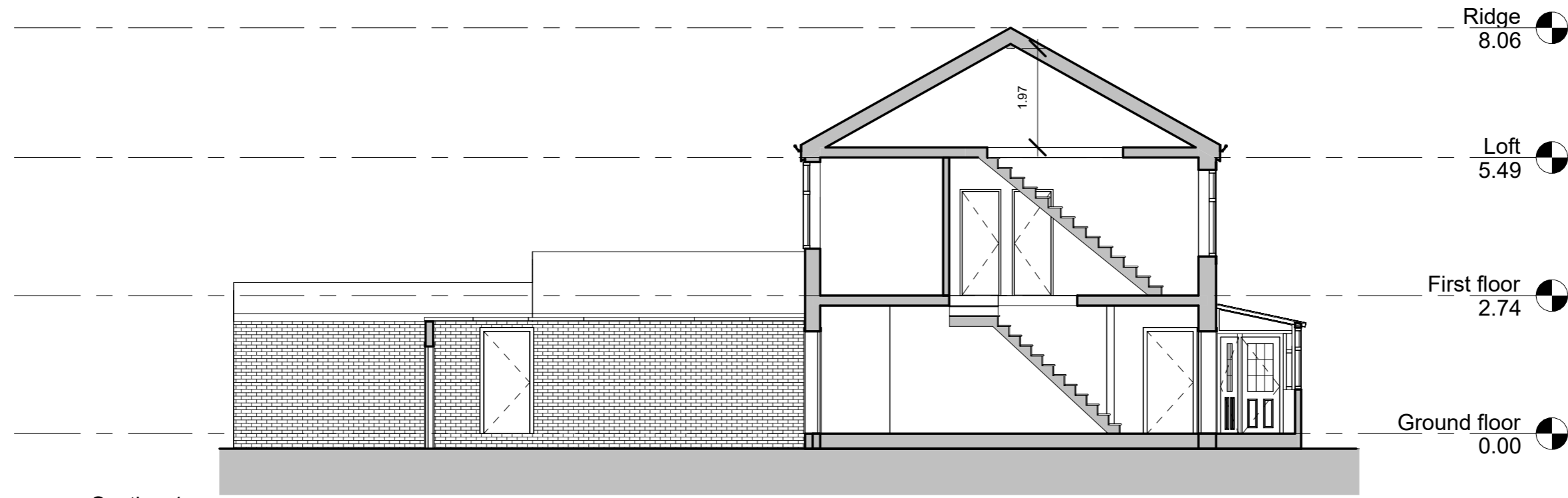
① Section 1 1 : 100
