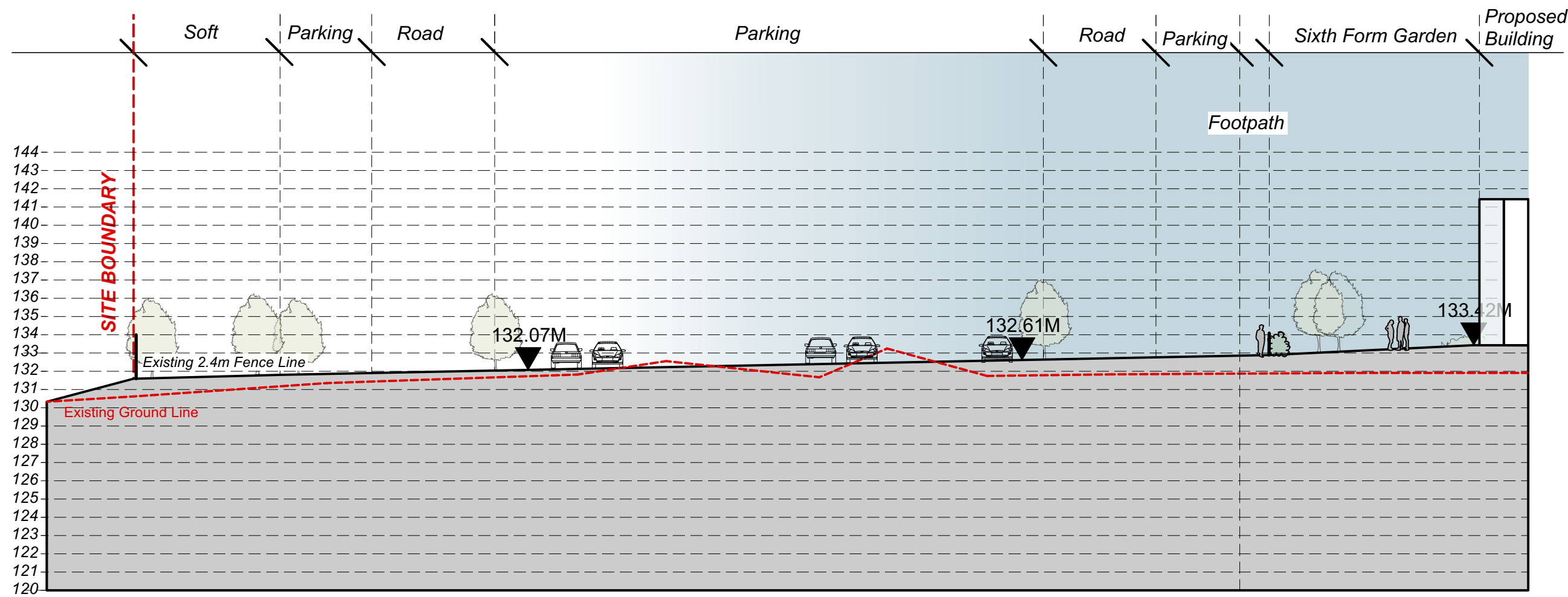
Site section C-C* Scale 1:250
