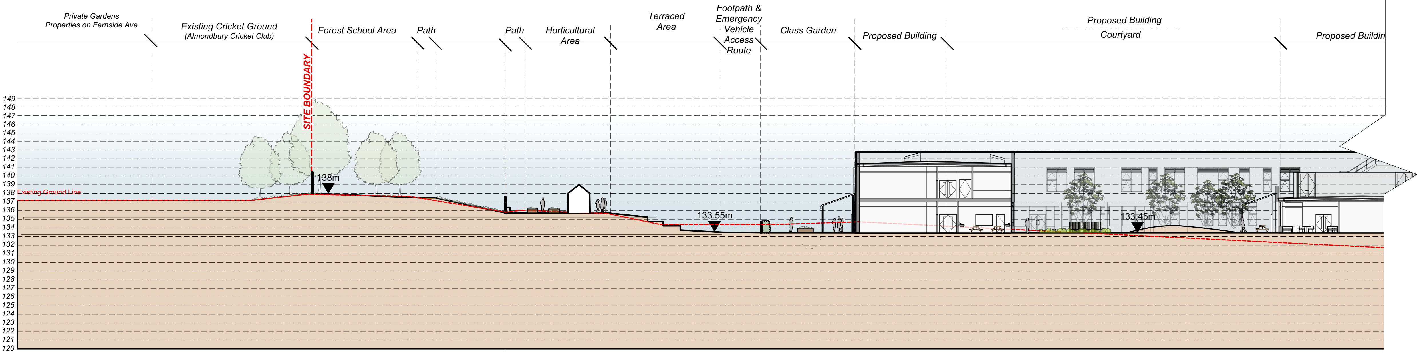
Site section B-B* Scale 1:250
