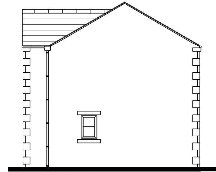
L.H side elevation 1:100
