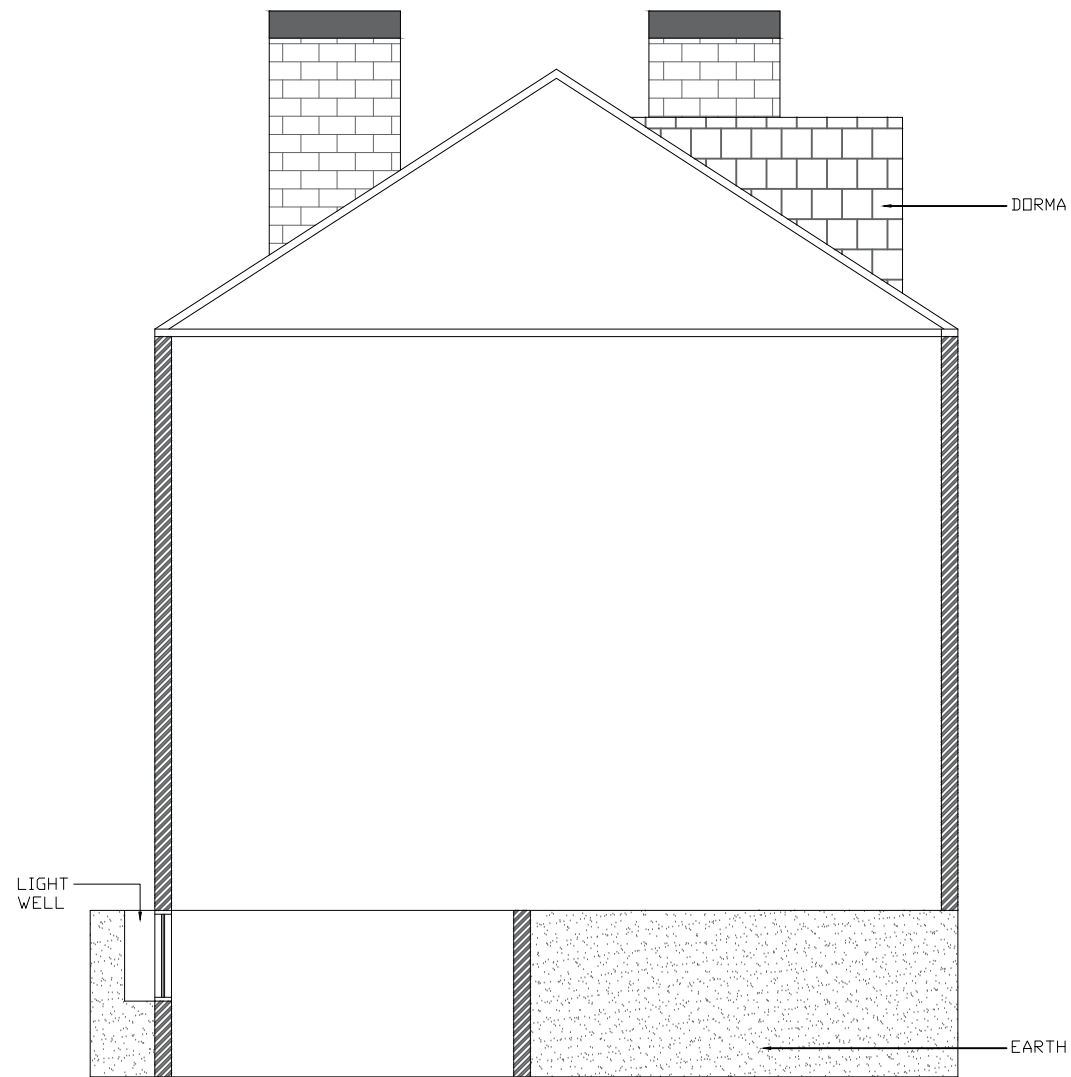
EAST SECTION SCALE: 1:100
