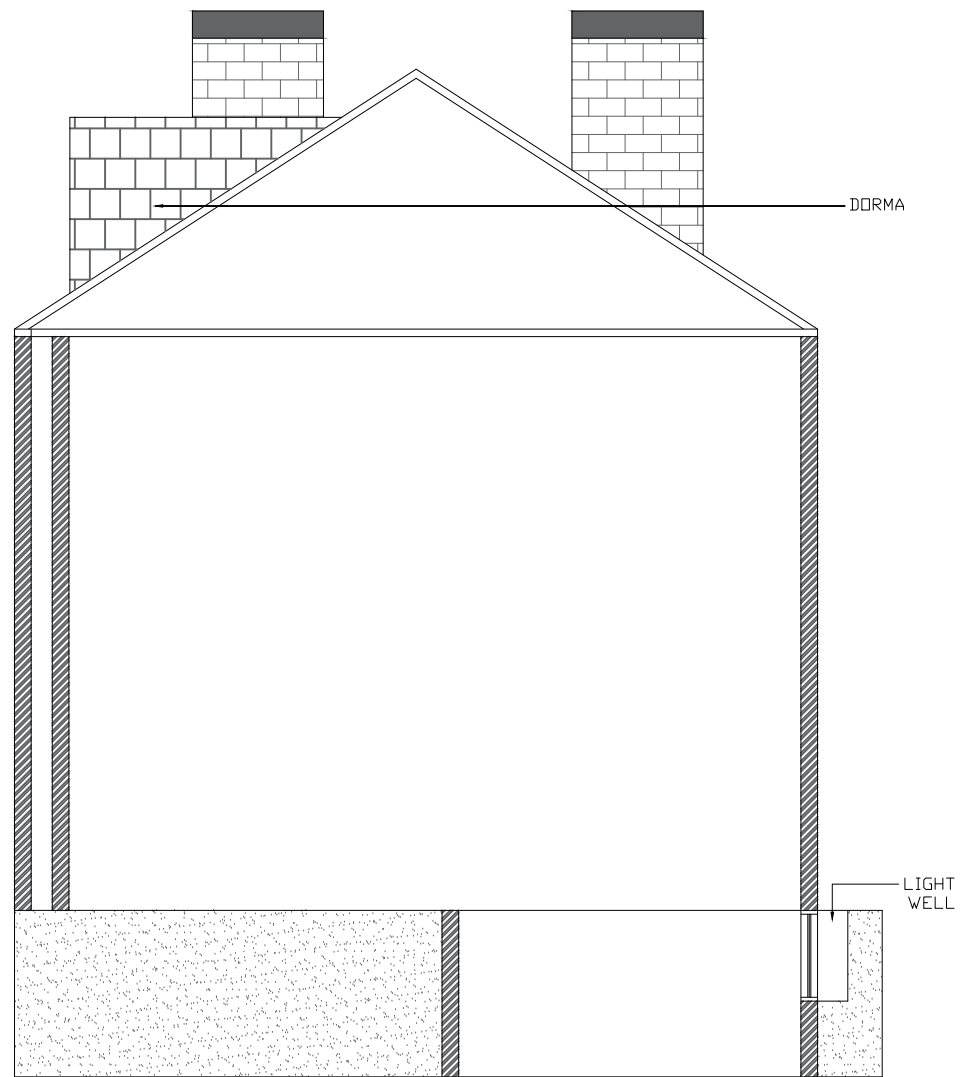
WEST SECTION SCALE: 1:100
