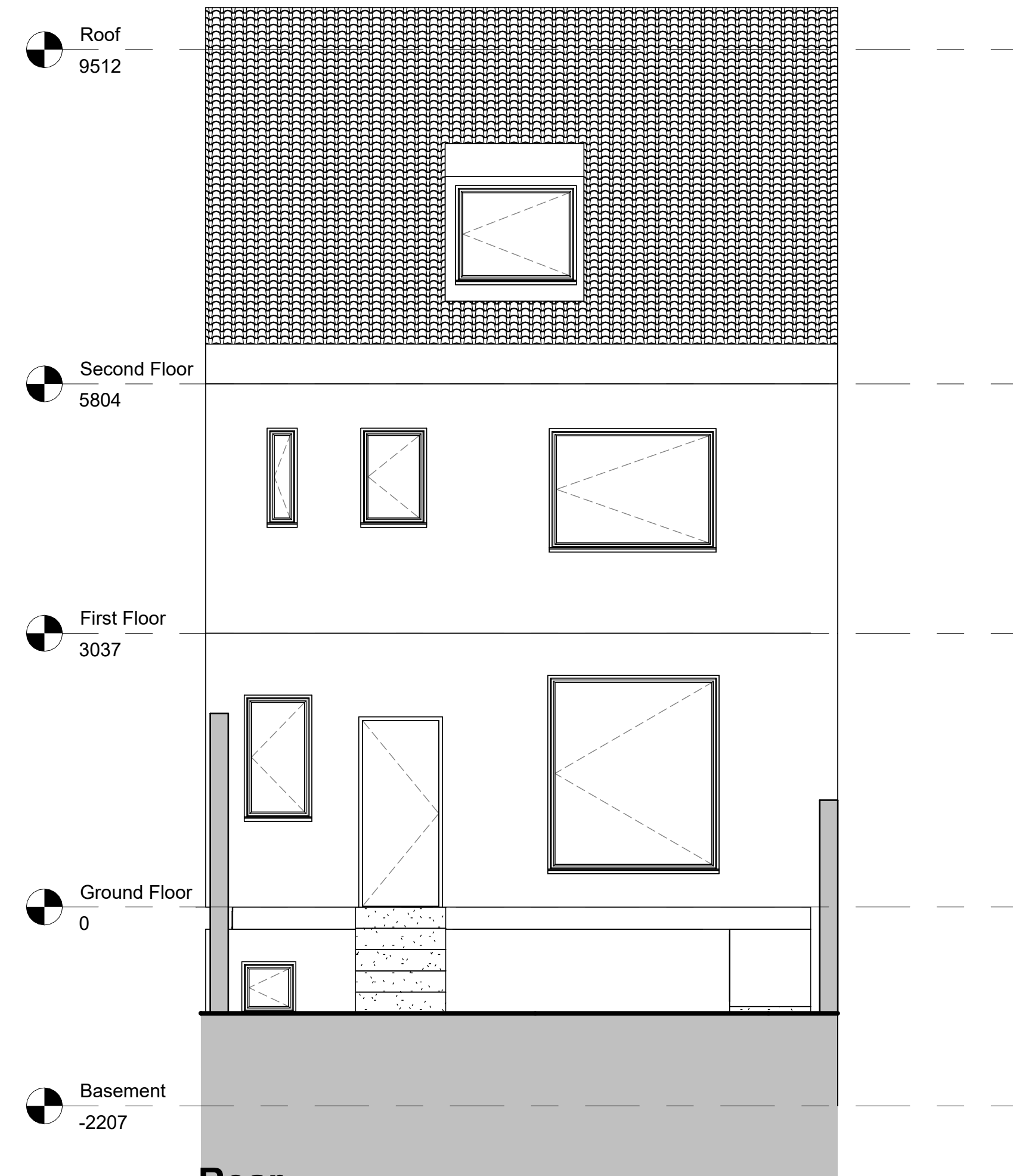
Rear 1 : 50
