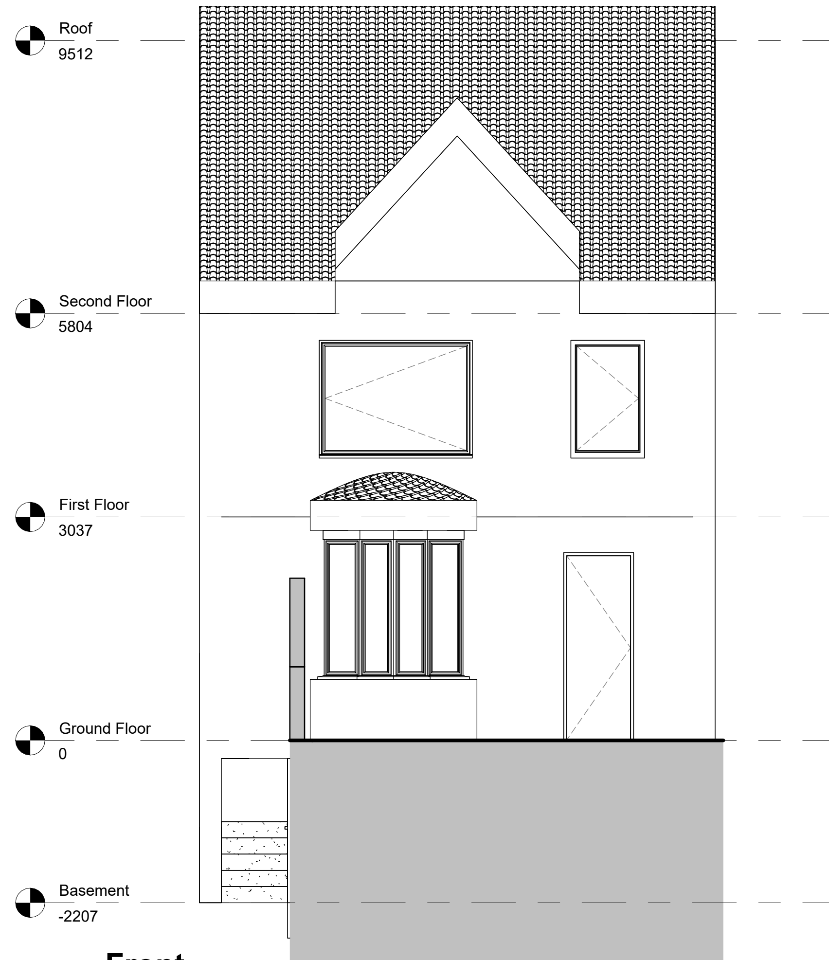
Front 1 : 50
