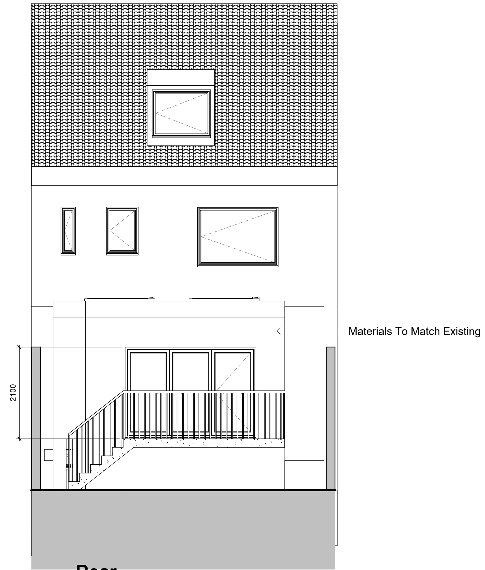
Rear 1 : 50
