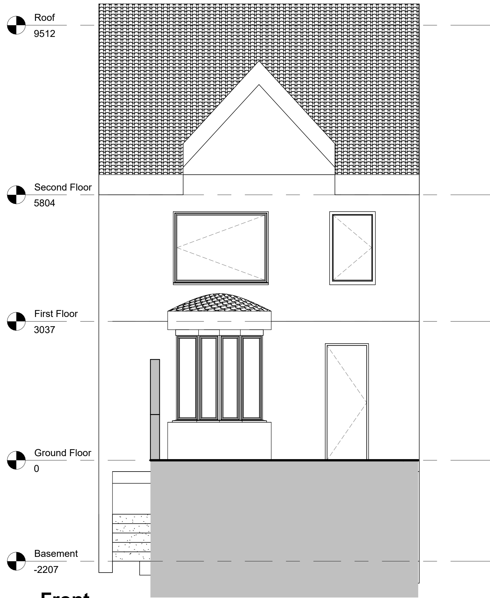
Front 1 : 50
