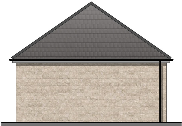
L.H.S. Elevation
