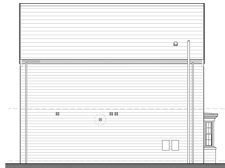
L.H.S. Elevation
