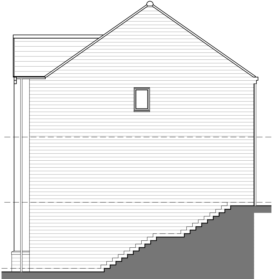
R.H.S. Elevation
