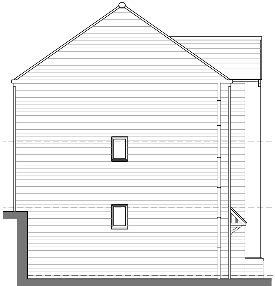
L.H.S. Elevation
