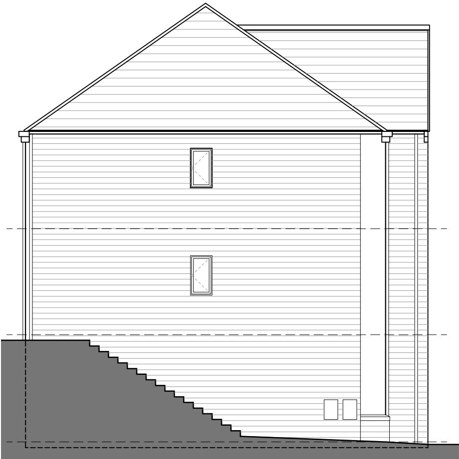
L.H.S. Elevation
