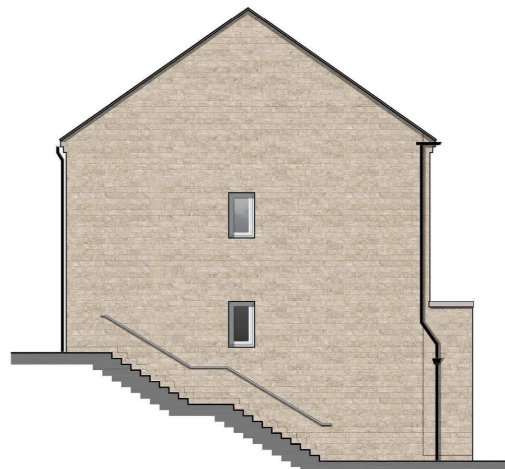
L.H.S. Elevation
