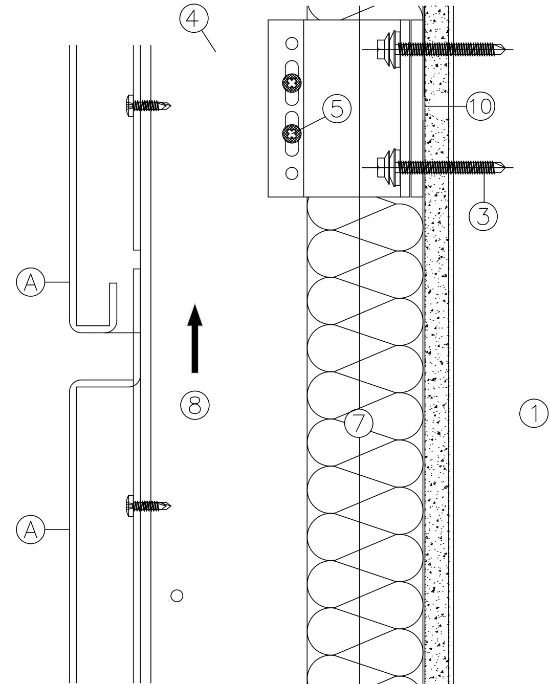
VERTICAL SECTION - RF1
