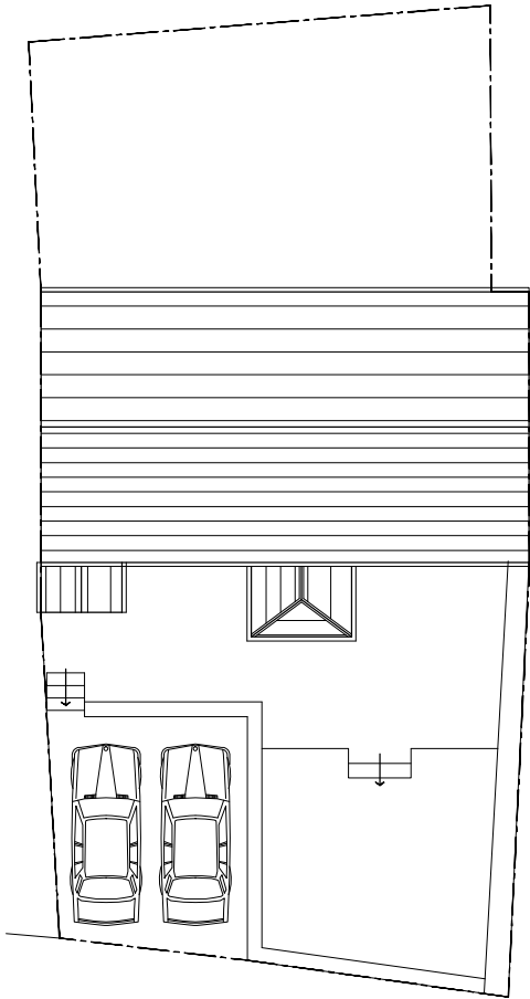
Site Plan 1:200
