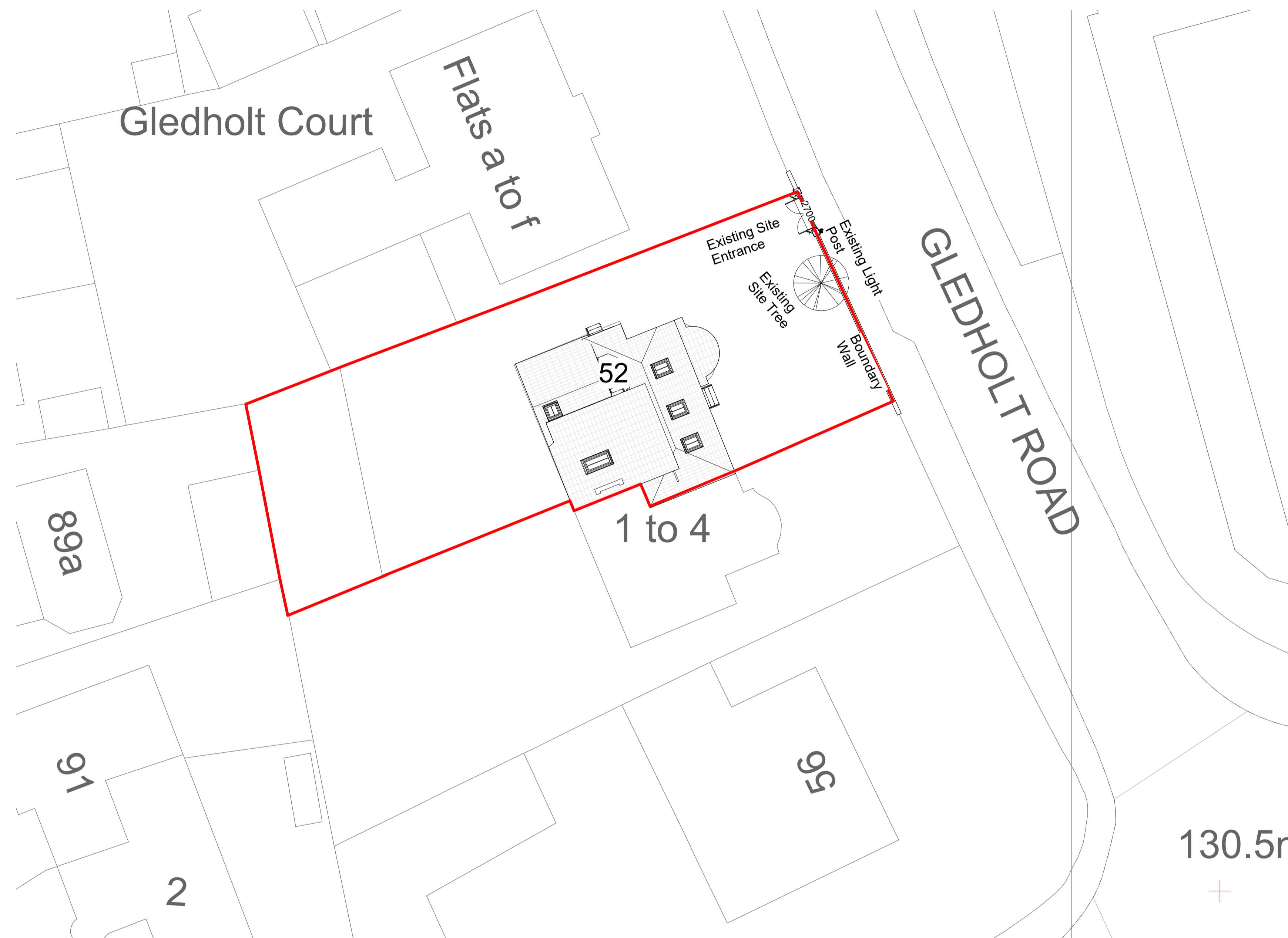
Site Plan 1 : 200
