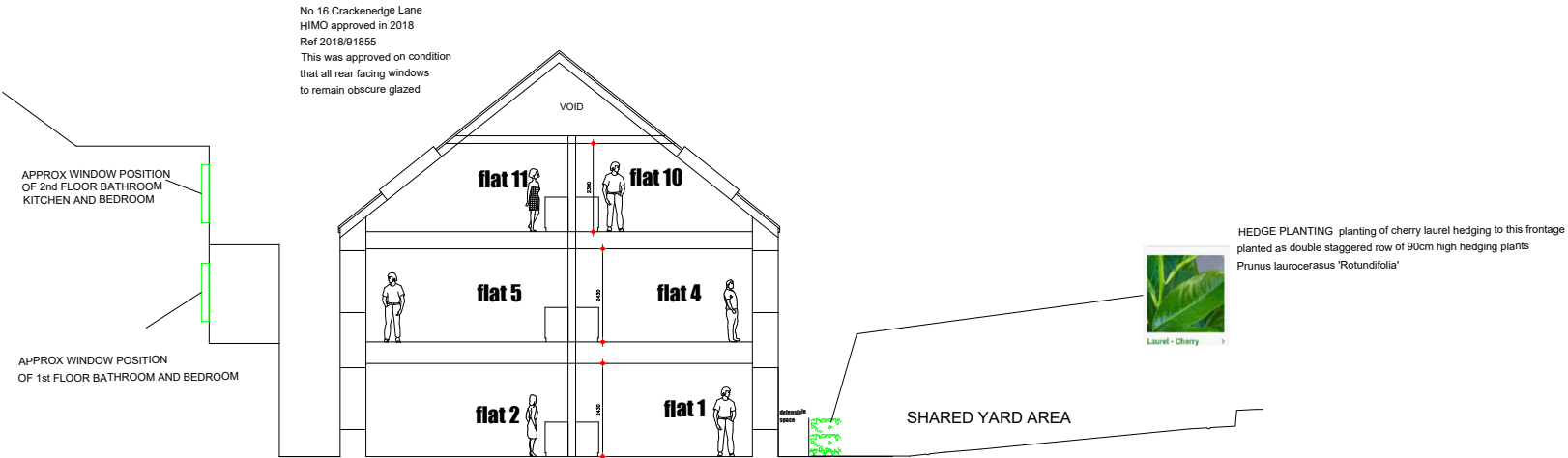
section a-a
