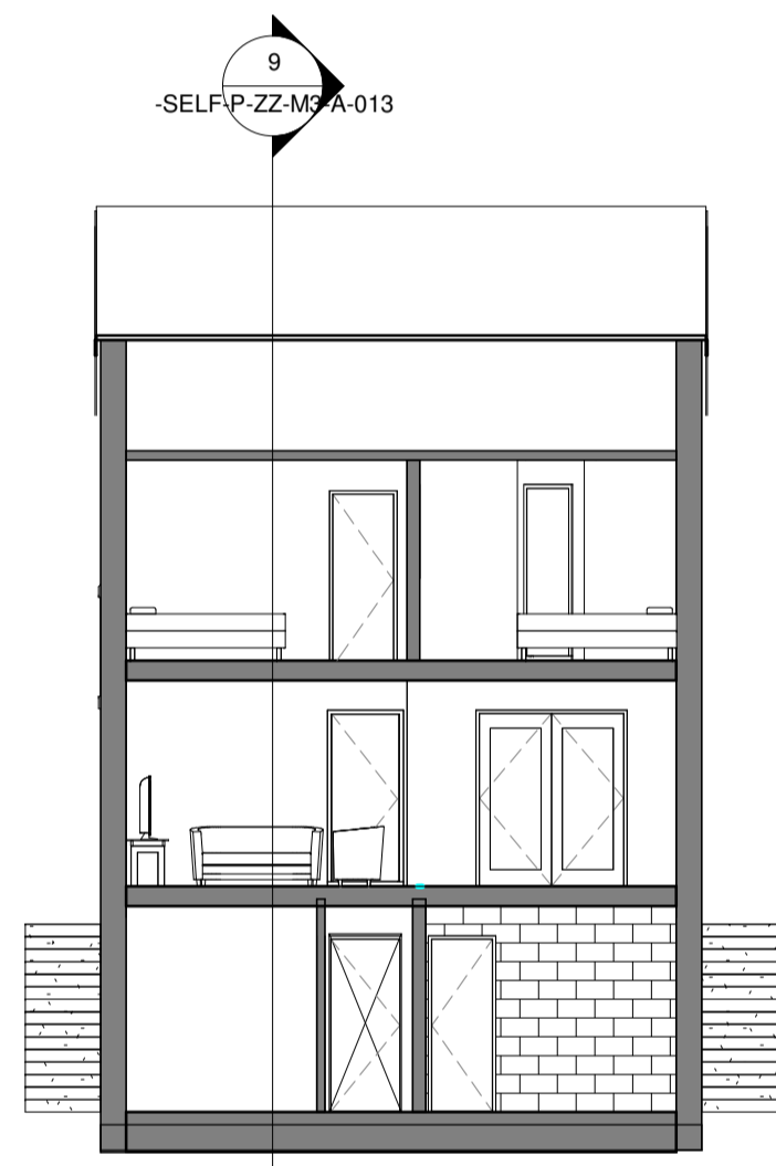
Section B - B 1 : 100
