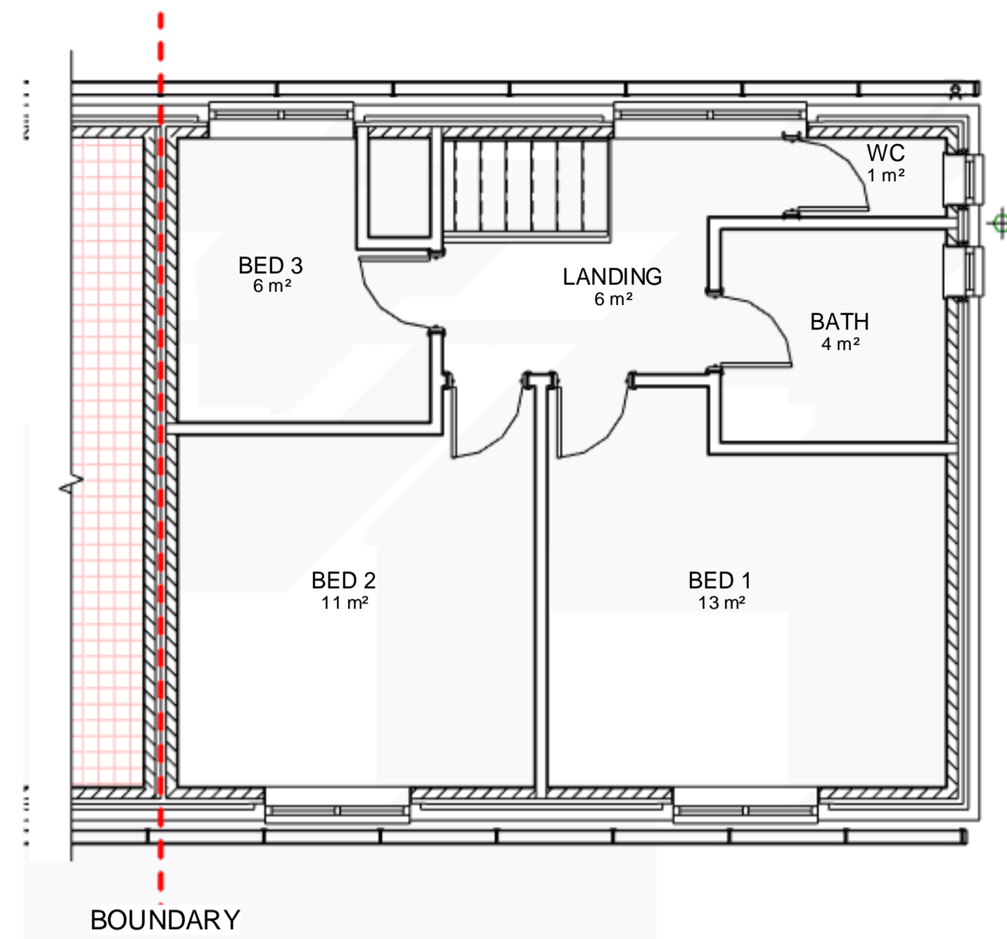
2 FF EXISTING 1 : 50
