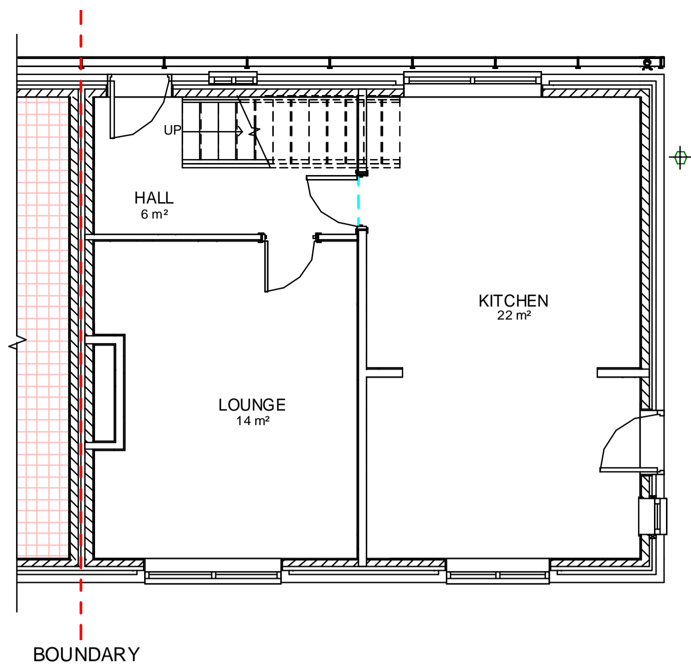
1 GF EXISTING 1 : 50
