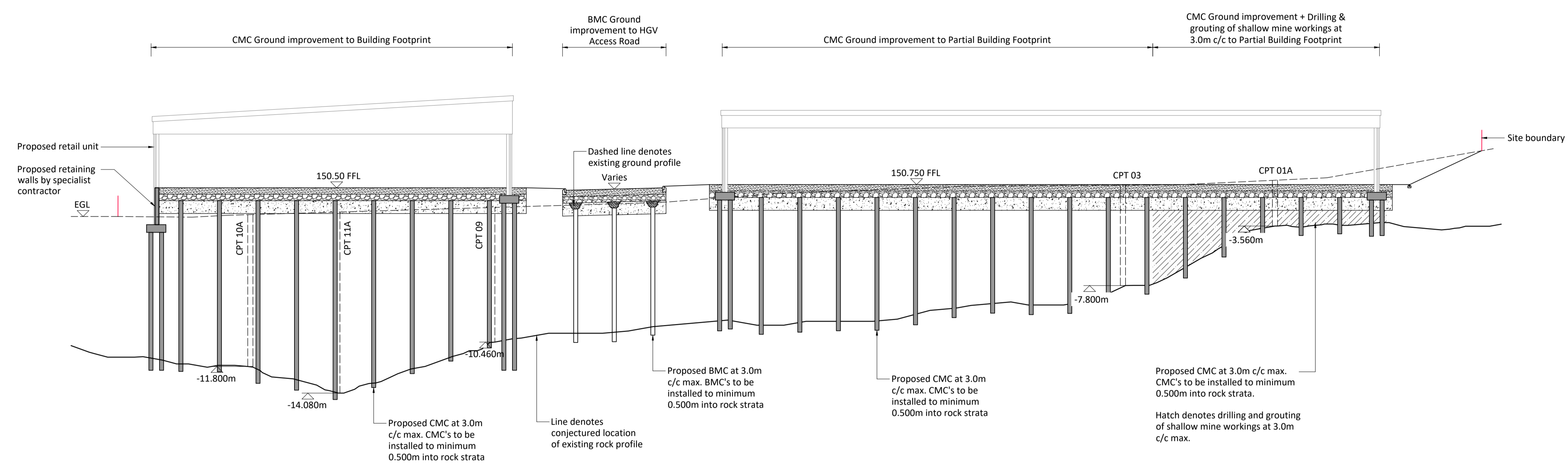
Section A-A Scale 1:200
