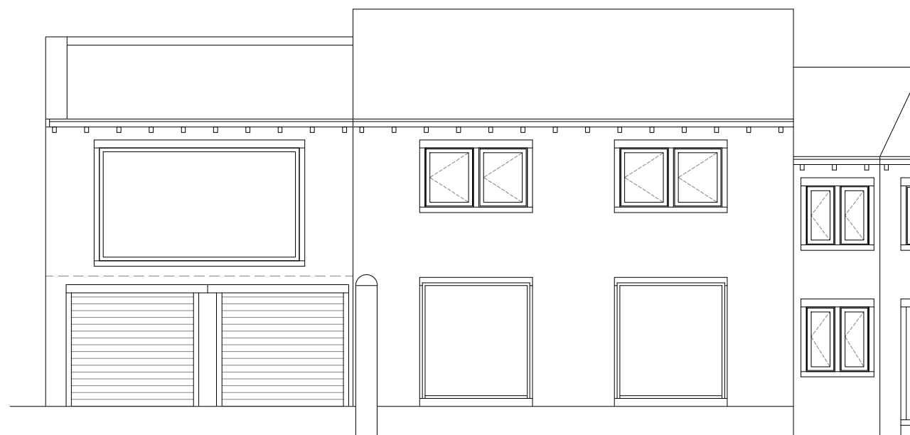
Elevation 01
