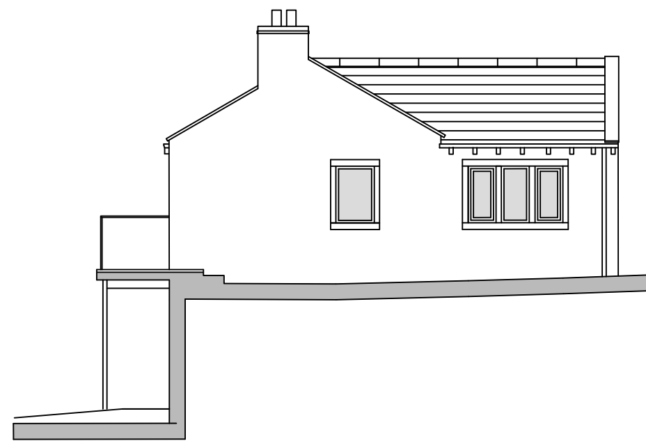
NE ELEVATION
