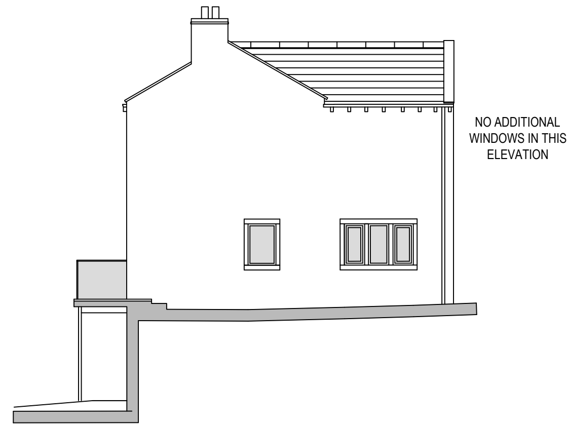
NE ELEVATION
