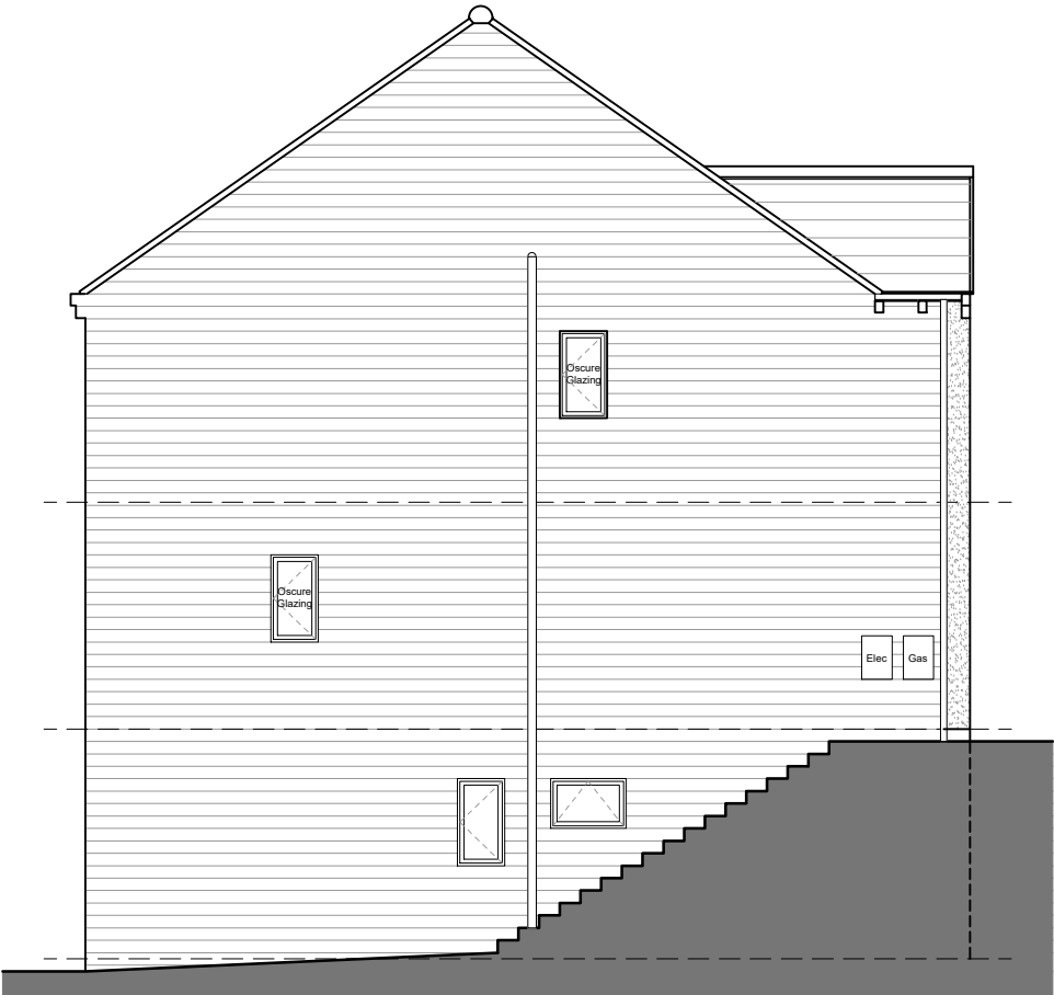
L.H.S. Elevation
