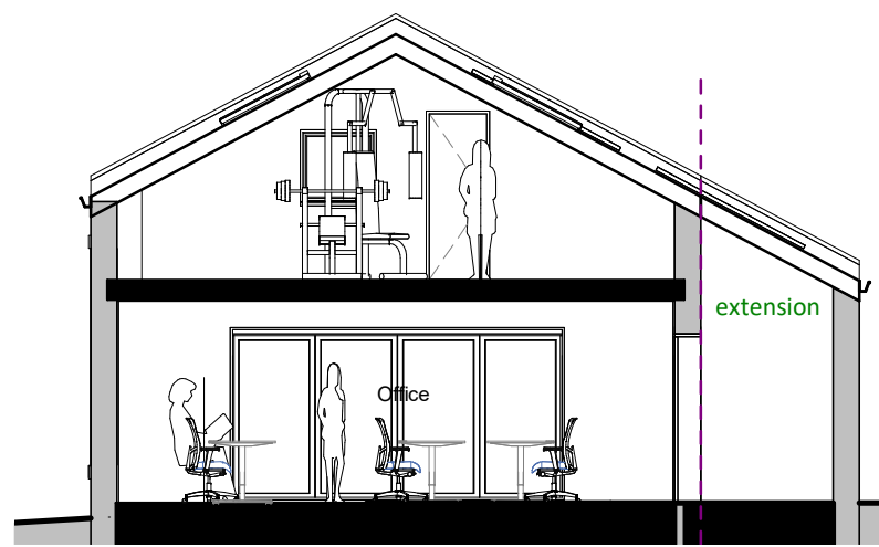
Section 2 1 : 100
