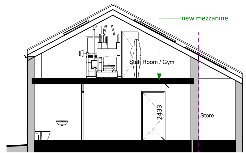
Section 1 1 : 100
